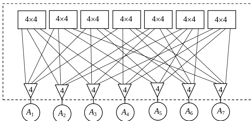
РИС. 2. Расширенная сеть PC(7,4,2)
