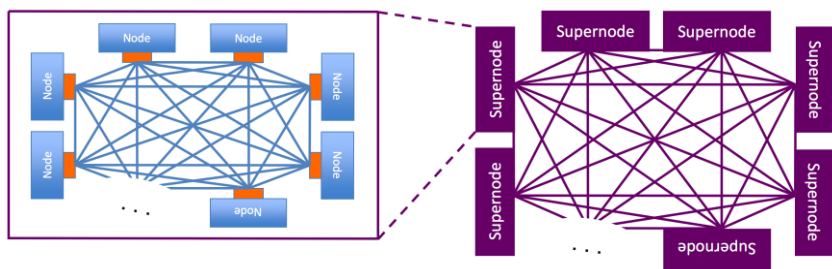
Рис. 1. Структура системной сети суперкомпьютера Blue Waters
