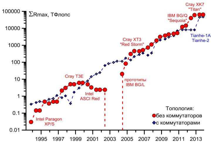
Рис. 4. Суммарная вычислительная мощность систем Rmax с коммутаторной и безкоммутаторной топологиями среди систем верхней десятки списка Top500
