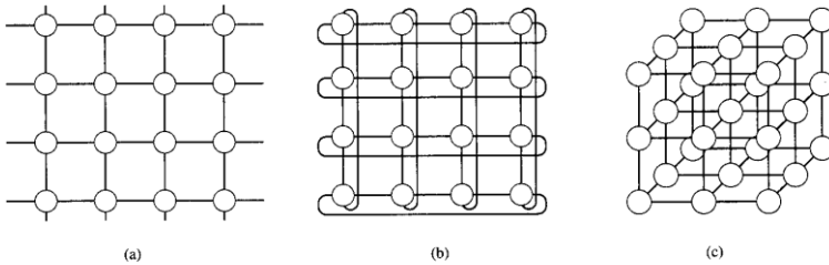
Рис. 3. Схема объединения узлов в топологии решетка и тор (a — решетка, b — 2-х мерный тор, c — 3-х мерная решетка)
