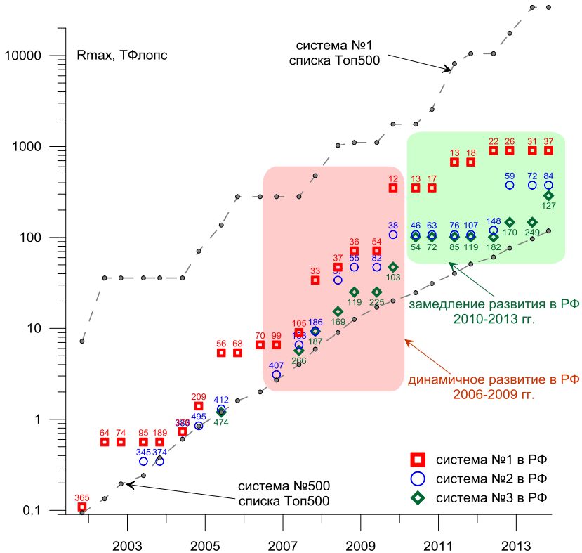
Рис. 1. Максимальная производительность лидирующих суперкомпьютеров согласно данным списка Top500 в 2001–2013 гг.
