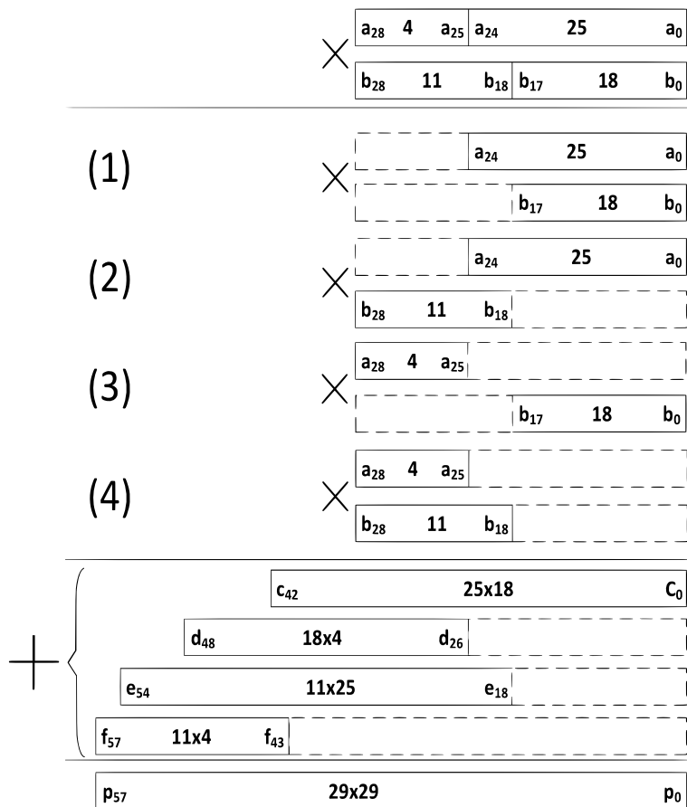
Рис. 1. Реализация умножения 29 \times 29 на умножителях 25 \times 18
