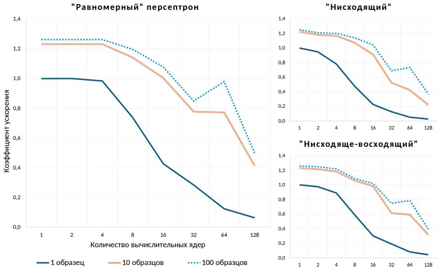
Рисунок 3. Эффективность выполнения задачи прямого распространения на одном ядре ПИВС с разным числом ядер для различных структур многослойного персептрона и различных размеров пакетов
