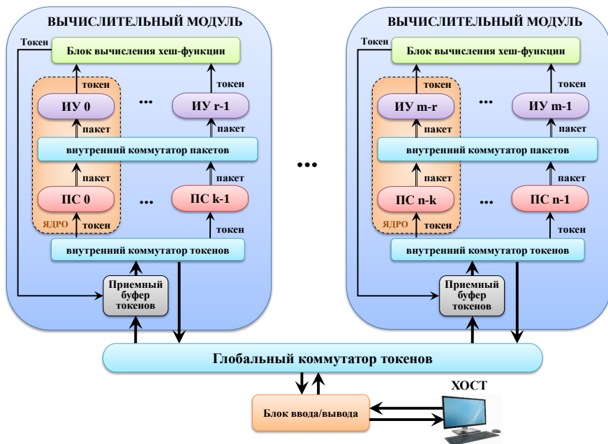
Рисунок 1. Архитектура параллельной потоковой вычислительной системы «Буран»
