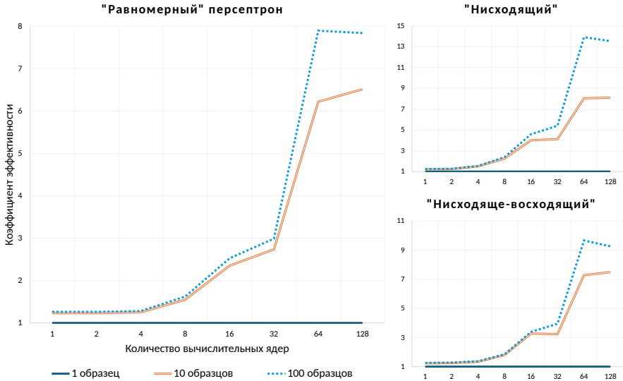
Рисунок 4. Эффективность «пакетного» выполнения задачи прямого распространения на ППВС для различных структур многослойного персептрона
