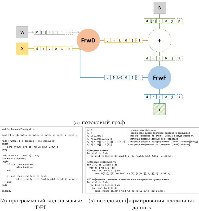
Рисунок 2. Алгоритм прямого распространения
