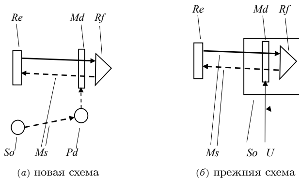
Рисунок 2. Оптический ретранслятор сети
