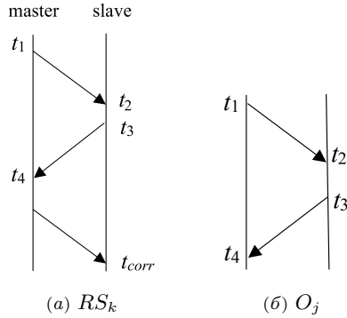
РИСУНОК 6. Измерение времени в RTP и вариант его использования в статье
