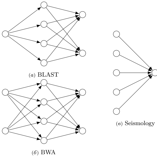
Рисунок 3. Примеры структур графов
