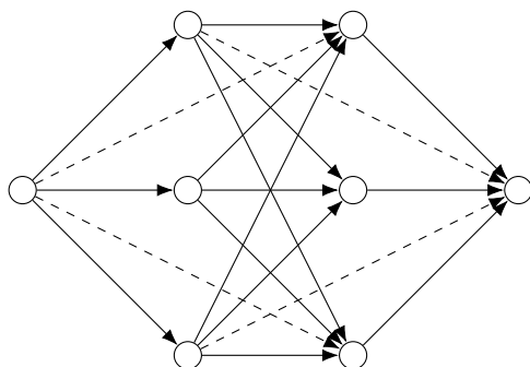
РИСУНОК 2. Граф, приближённо удовлетворяющий определению многостадийного графа с однородными зависимостями
