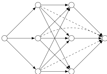
Рисунок 1. Пример многостадийного графа с однородными зависимостями. Сплошные стрелки обозначают зависимости между соседними стадиями, а пунктирные стрелки обозначают зависимости между несоседними стадиями.
