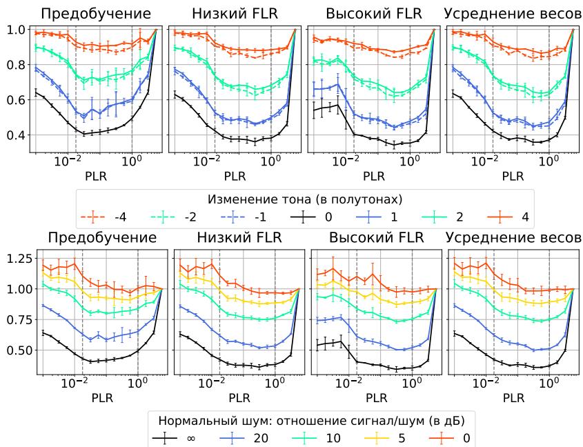
Рисунок 7. WER на тесте при применении различных аугментаций
