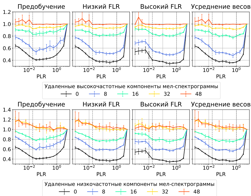
Рисунок 8. WER на тесте при маскировании компонент мел-спектрограммы
