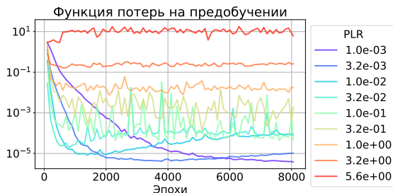
Рисунок 1. Функция потерь CTC
