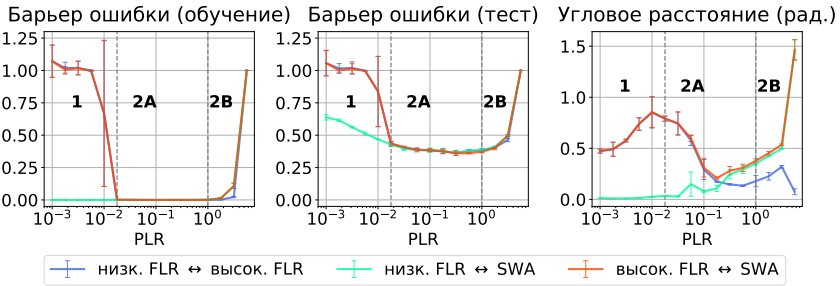
Рисунок 5. Геометрия пространства весов между решениями, полученными с низким FLR = 10^{-3} , высоким FLR = 3.2 \cdot 10^{-2} и SWA из 5 моделей. Вертикальные пунктиры проведены по крайним значениям PLR, отнесенным к подрежиму 2A: слева от левого пунктира лежит режим 1, справа от правого – подрежим 2B. Угловое расстояние вычисляется в радианах. Показаны среднее и стандартное отклонение по трем запускам.
