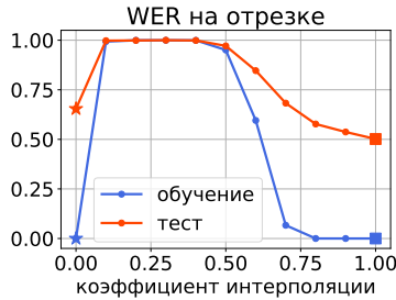
Рисунок 4. Пример интерполяции в пространстве весов между двумя моделями, обученными с низким \text{FLR} = 10^{-3} (левый конец, звезда) и высоким \text{FLR} = 3.2 \cdot 10^{-2} (правый конец, квадрат). Обе модели получены предобучением с \text{PLR} = 10^{-3} .
