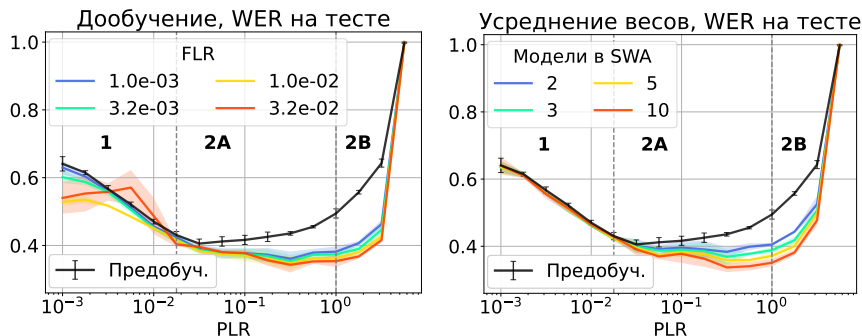
Рисунок 3. WER после дообучения и усреднения весов алгоритмом SWA: черная линия показывает качество после предобучения, вертикальные пунктиры проведены по крайним значениям PLR, отнесенным к подрежиму 2А.
