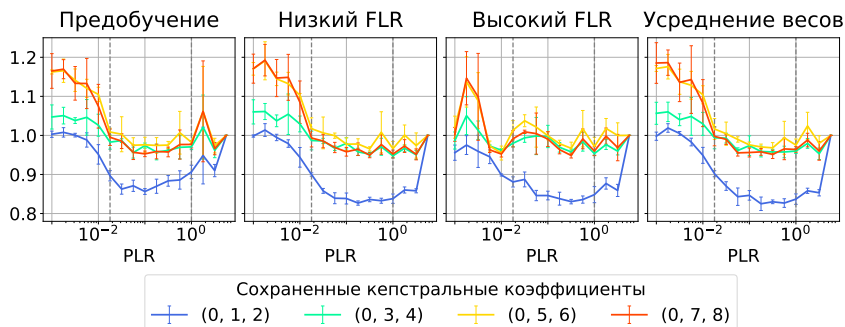
Рисунок 6. WER на тесте для различных компонент мел-частотного кепстра
