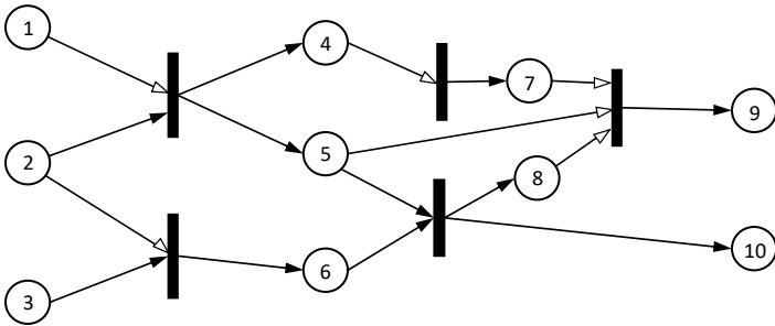
Рисунок 2. Пример вычислительного графа. Т-вершины пронумерованы и показаны кружочками, А-вершины полосками. Стрелка (из t в a ) имеет белый конец, когда она стирающая, то есть когда M(t, a) = \text{false} , иначе – черный.
